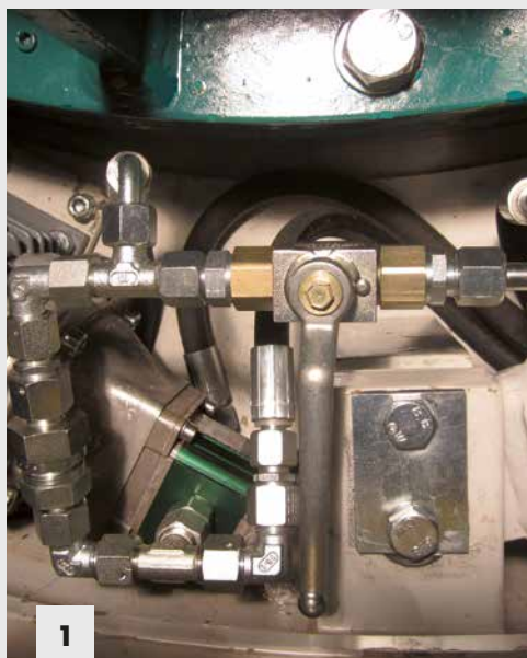
Fig. 1: Le rotor lui-même est équipé d'un groupe hydraulique autonome pour le réglage des couteaux. Une pompe hydraulique entraînée par un moteur électrique produit la pression requise pour le réglage des couteaux.
